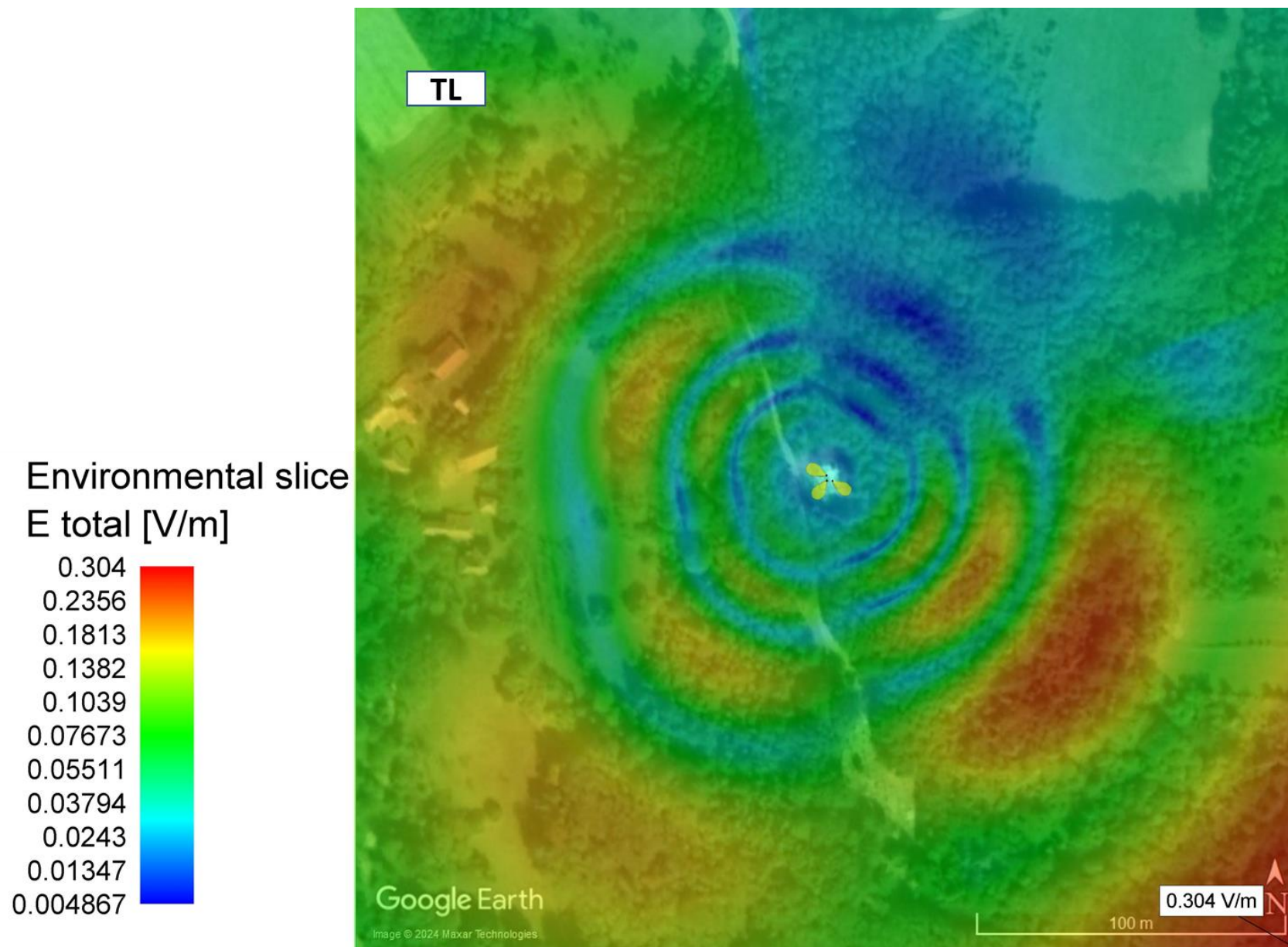
Слика 4.3. Јачина електричног поља на тлу када радио-систем LTE800 оператора А1 Србија ради максималним капацитетом
